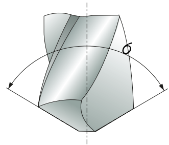
Bild 7. Spitzenwinkel \sigma Figure 7. Point angle \sigma
