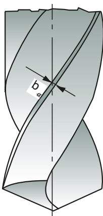
Bild 3. Fasenbreite b_\alpha Figure 3. Margin width b_\alpha
