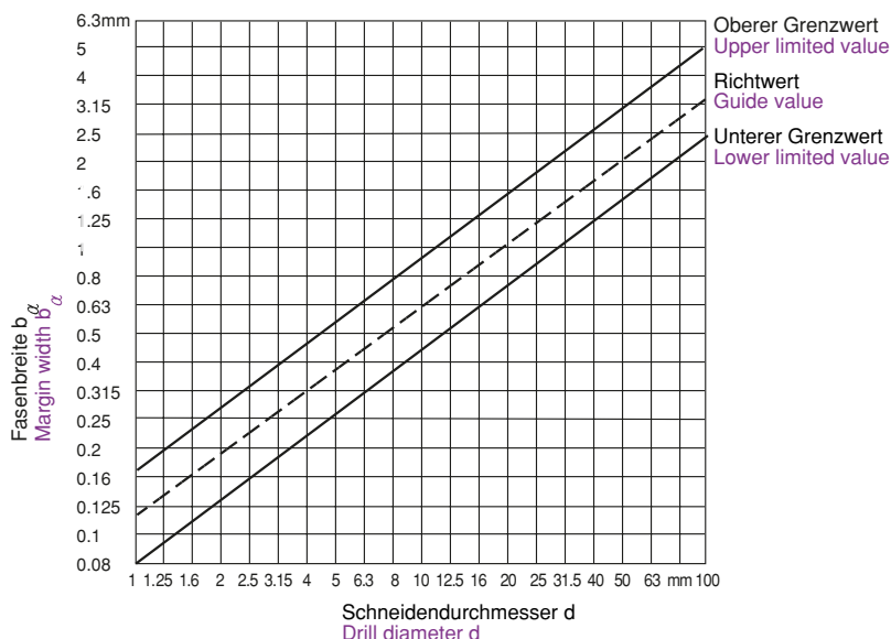
Bild 4. Fasenbreite b_\alpha Figure 4. Margin width b_\alpha
