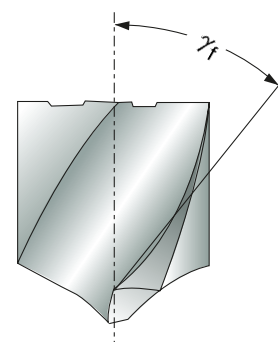
Bild 6. Seitenspanwinkel \gamma_f Figure 6. Side rake angle \gamma_f
