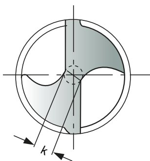
Bild 1. Kerndicke k Figure 1. Web thickness k
