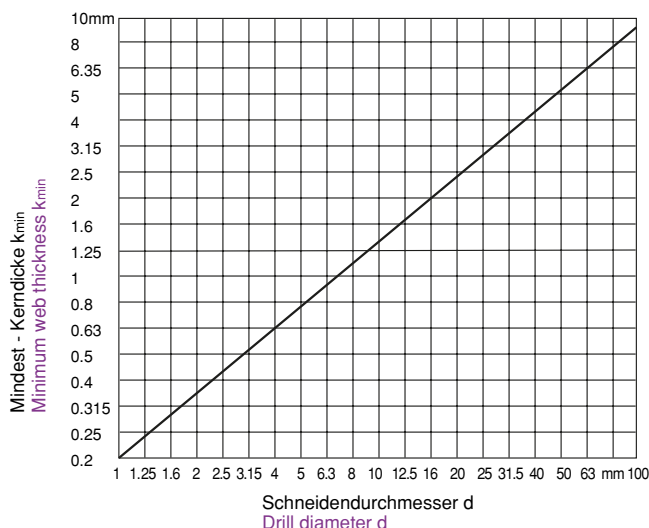
Bild 2. Kerndicke k_{\min} Figure 2. Web thickness k_{\min}
